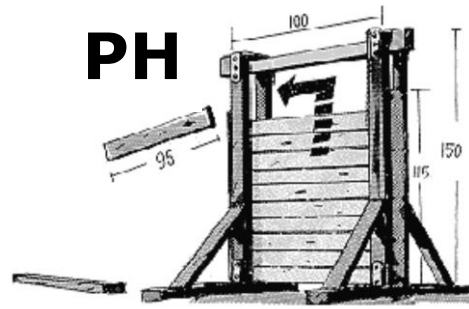
Bild 2. Plankhinder PH
