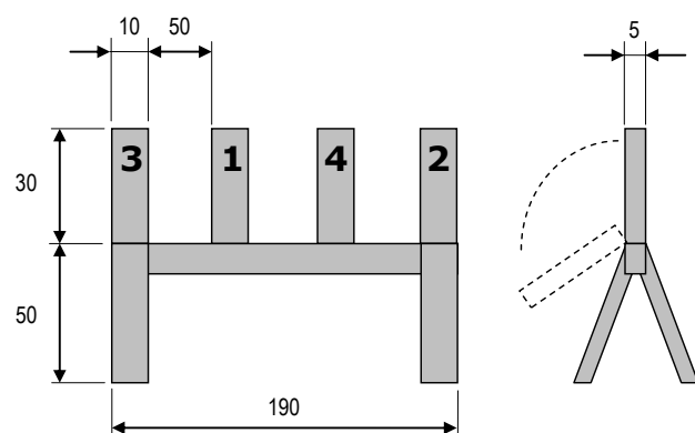
Bild 7. Klaffhinder KH
