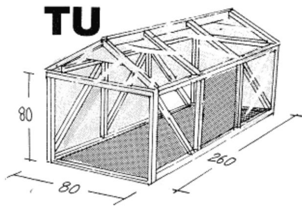
Bild 4. Tunnel TU
