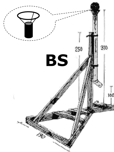
Bild 5. Bollställning BS
